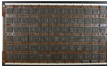
(processeur de Cray 1)
